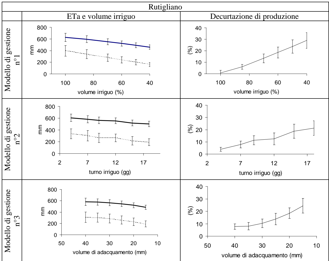
Figura 5. Rutigliano, barbabietola a semina autunnale: Evapotraspirazione effettiva (linea intera) e volume irriguo stagionale (linea tratteggiata) e decurtazione di produzione stimati con volumi irrigui sub-ottimali, con tre modelli di gestione irrigua.
