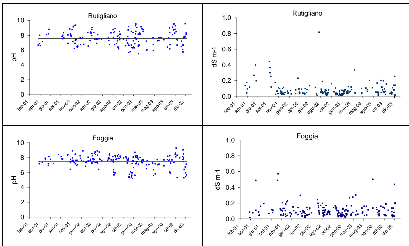
Figura 8 Valori di pH e di conducibilità elettrica (CE in dS m -1 ) misurati in campioni di acqua piovana a Foggia e a Rutigliano.
