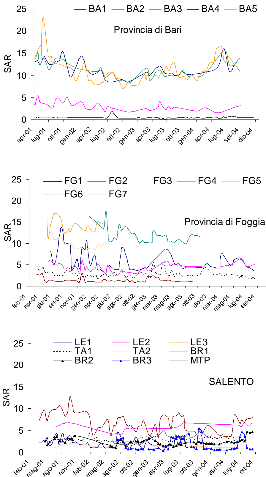
Figura 7. Variazioni di SAR dell'acqua di falda, misurata durante il periodo aprile 2001 – dicembre 2004, in 21 siti di campionamento
